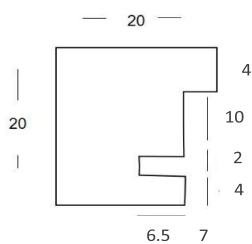
Querschnitt
