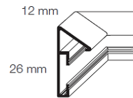
Profil 173
