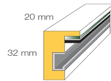
Profil 20/32
