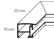
Profil 30
