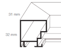
Profil 72
