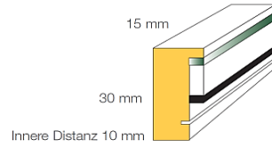
Profil A30
