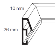
Profil 170
