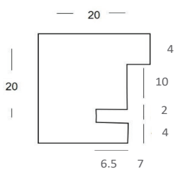
Querschnitt
